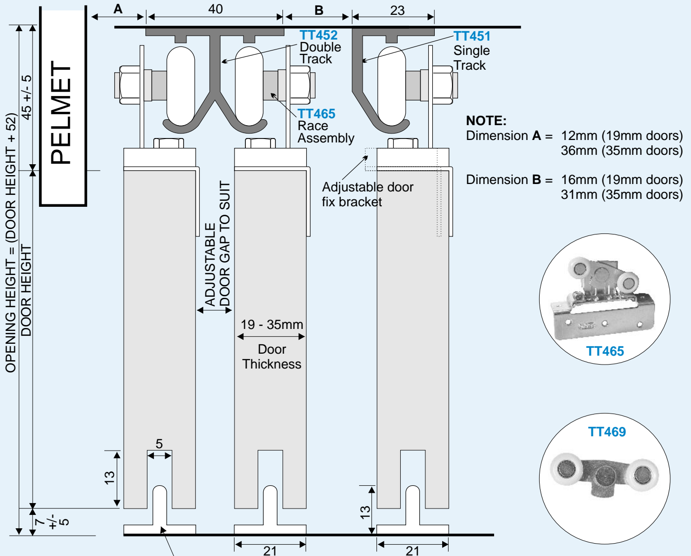
TT30 DOOR GUIDE
